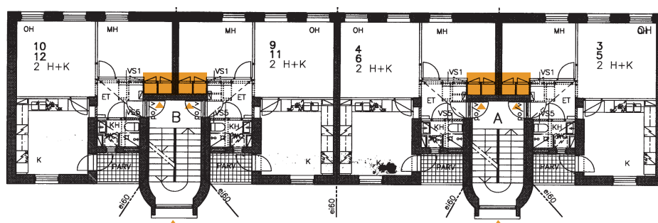
TYYPPI 6 Kansanasuntojen asuinrakennukset A4 ja A5 (Kuvassa yllä pohjapiirustus rakennuksesta A5, 2-3 krs., peruskorjauksen pohjapiirustus vuodelta 2001)
